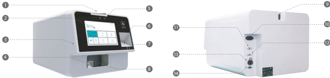
1. Entrée de pièces, 2. Écran tactile, 3. Porte de la machine, 4. Sortie de pièces, 5. Voyant indicateur pour le validateur de pièces actif, 6. Entrée et sortie de billets, 7. Voyant indicateur pour le validateur de billets actif, 8. Serrure cachée pour ouvrir la porte, 9. Bouton marche / arrêt de la machine (ON / OFF), 10. Connecteur câble d'alimentation, 11. Connecteur de câble OTG, 12. Connecteur de câble USB, 13. Connecteur Ethernet, 14. Connecteur de service RS232.
